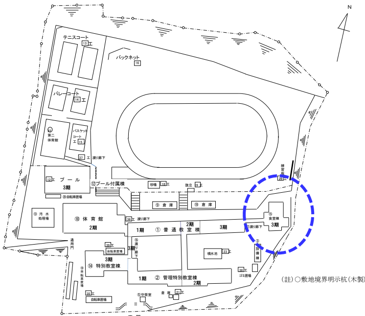
大阪府立槻風館高等学校配置図
